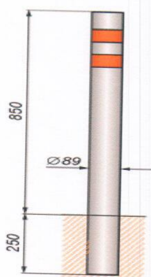
Рис. 4. Внешний вид и размеры столбика ограждения
