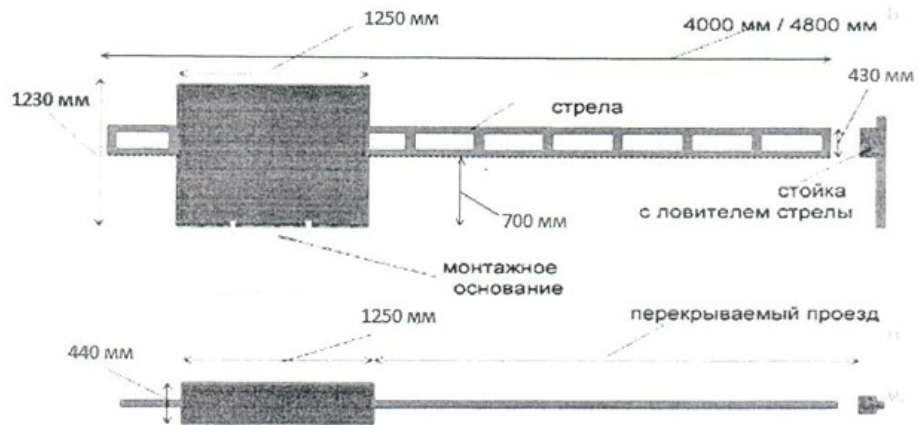
Рис. 2 Размеры шлагбаума
