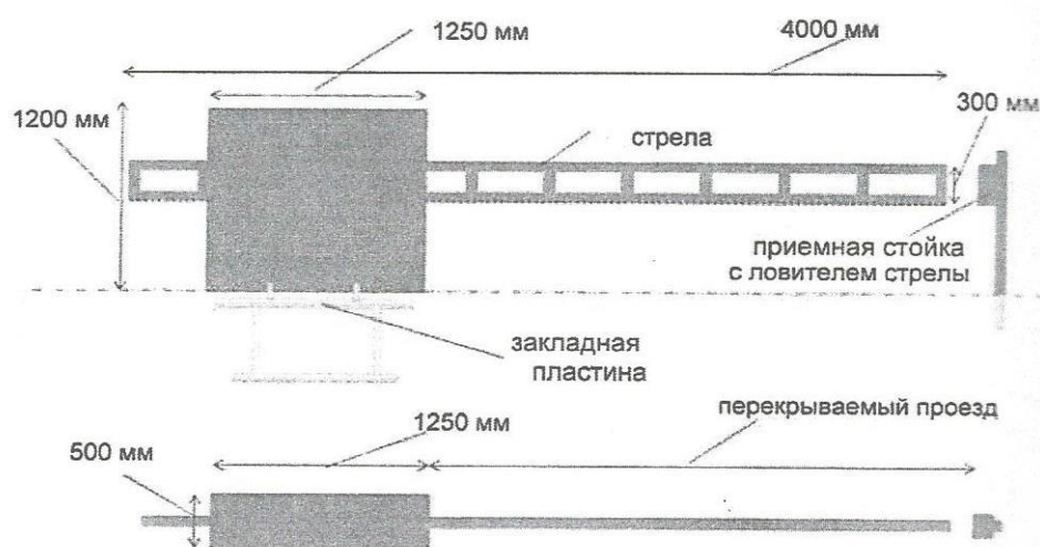
Рис. 2. Габаритные размеры
