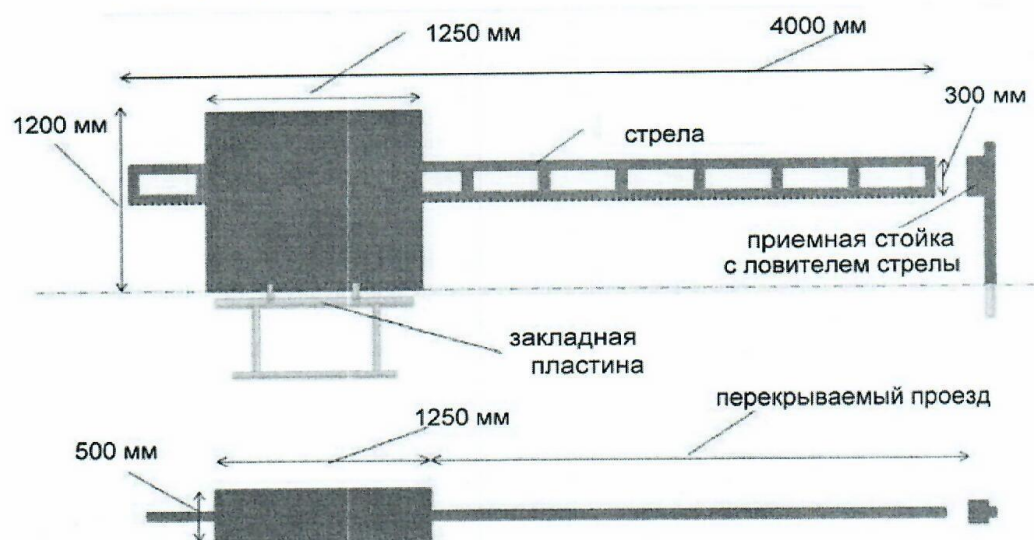
Рис. 2. Габаритные размеры
