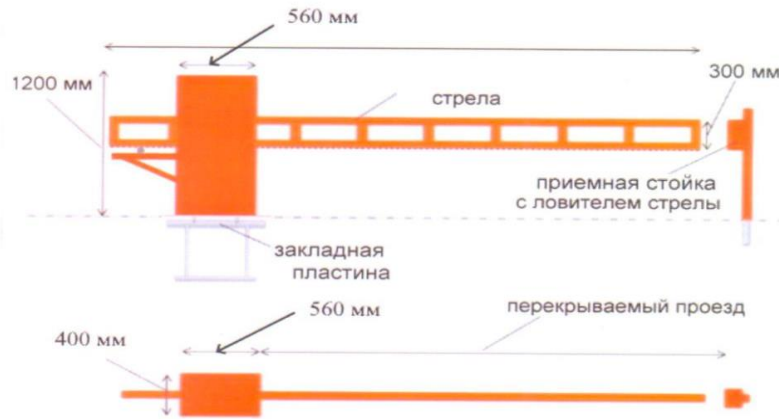
Рис. 2. Габаритные размеры
